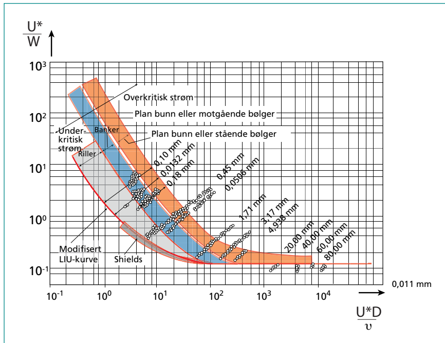
Figur 5.22 Betingelser for bunnformer, etter Simons & Richardson (1966).
