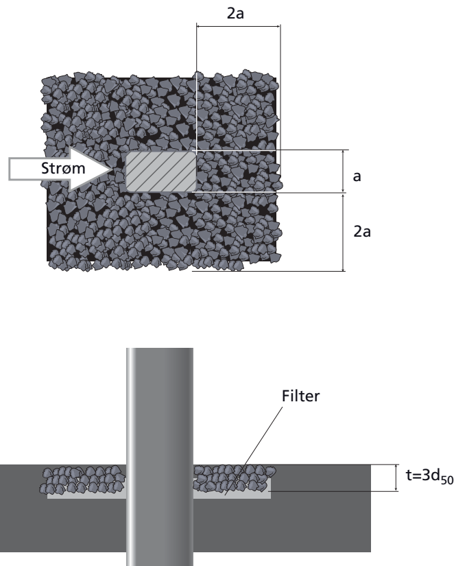
Figur 6.21 Sikring rundt brupilar (etter Lagasse 2006).
