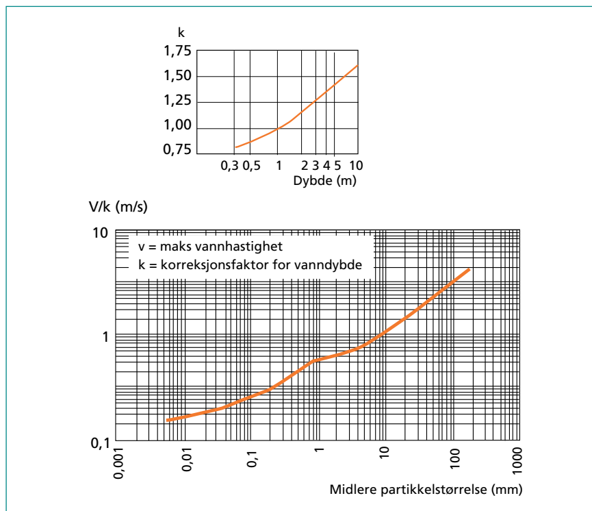
Figur 5.48 Praktisk dimensjonering av dekklag av vanlig stein, \rho_s = 2560 \text{ kg/} \text{m}^3 , på flat bunn. Bygger på forskrifter fra USA og tidl. USSR.
