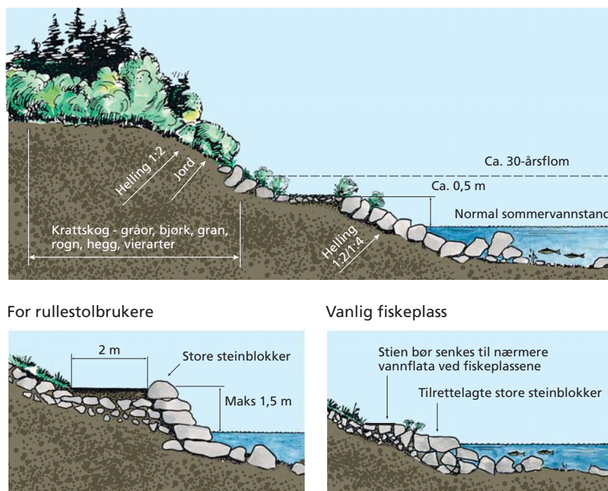
Figur 6.5 Erosjonssikret elvebredd med tekniske og miljømessige detaljer og tegning av fotgrøft og fiskeplass.
