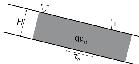
Figur 5.13 Skjærspenning langs bunnen ved normalstrømning.
