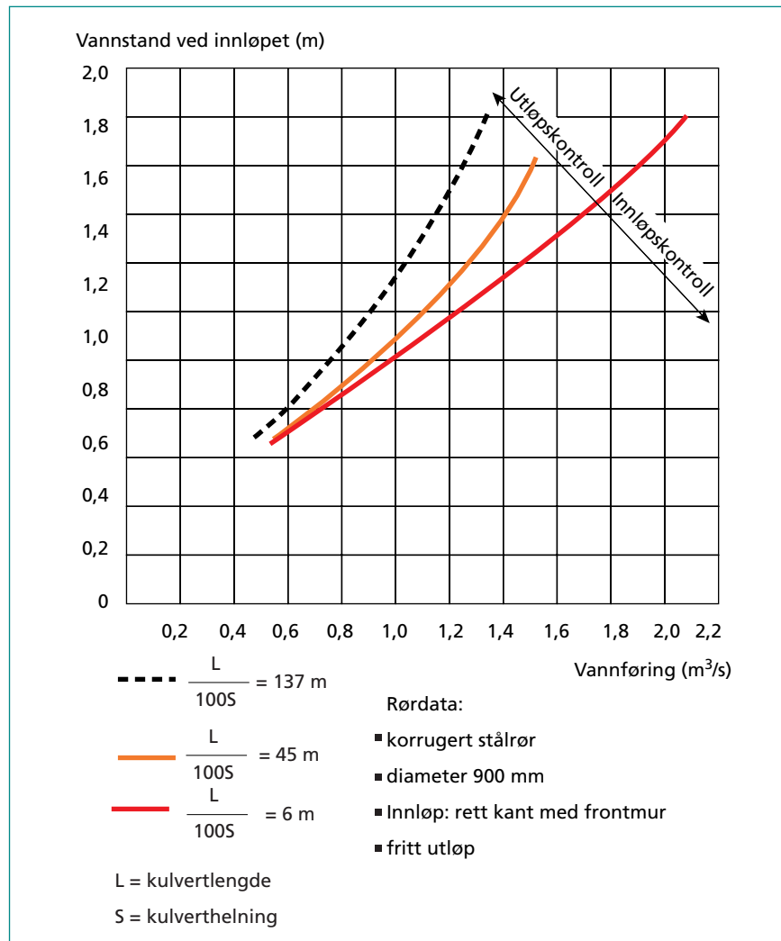
Figur 10.5 Kapasiteten til en kulvert med utløps- og innløpskontroll. Korrugert stålrør, D = 900 \text{ mm} .
