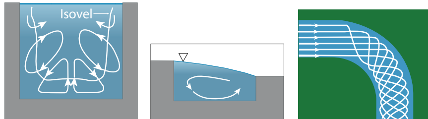
Figur 5.27 Sekundære strømmer i hjørner og i en sving.
