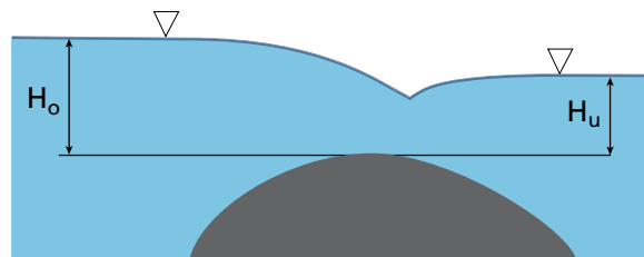
Figur 4.16. Grensen for fritt overløp.
