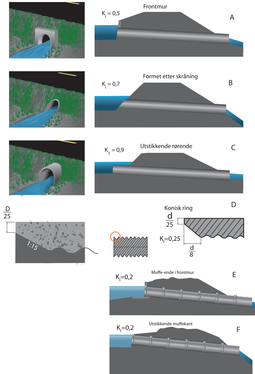
Figur 10.6 Skisse av innløpstyper for rørkulverter ( K_i = innløpstap, sml avsnitt 3.5.7).
