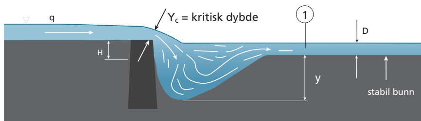
Figur 8.31 Prinsippskisse av terskel med erosjonsgrop.
