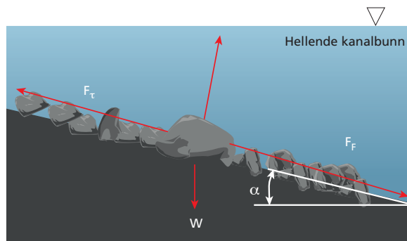
Figur 5.8 Krefter på korn i sideskråning og på hellende bunn. Definisjonsskisser.
