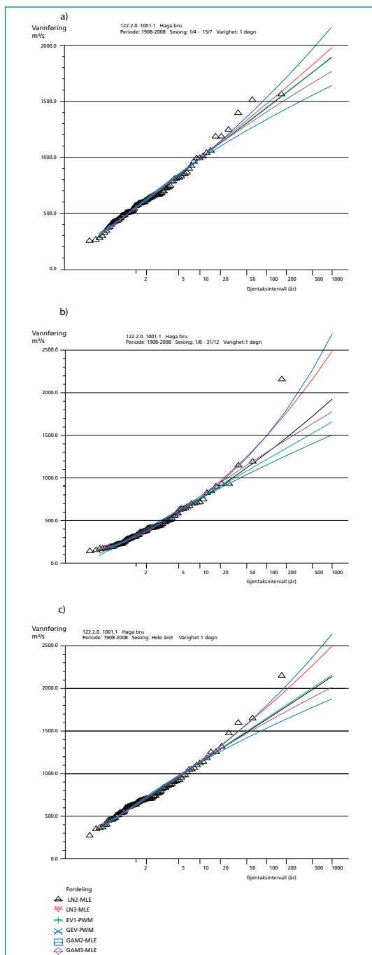
Figur 6. Eksempel på flomfrekvensanalyser av data fra målestasjonen 122.2 Høga bru. Stasjonen ligger i Gaula i Sør-Trøndelag og har bortimot 100 år med observasjoner.
