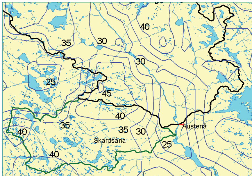
Figur 2. Utsnitt av avrenningskart for normalperioden 1961–90 for øvre del av Tovdalsvassdraget. Isohydater (avrenningskoter) er markert med blå linjer og er gitt i enheten l/s km 2 . På kartutsnittet er det en variasjon i avrenning fra 25 til 45 l/s km 2 med de laveste verdiene nær dalbunnen i hovedvassdraget.
