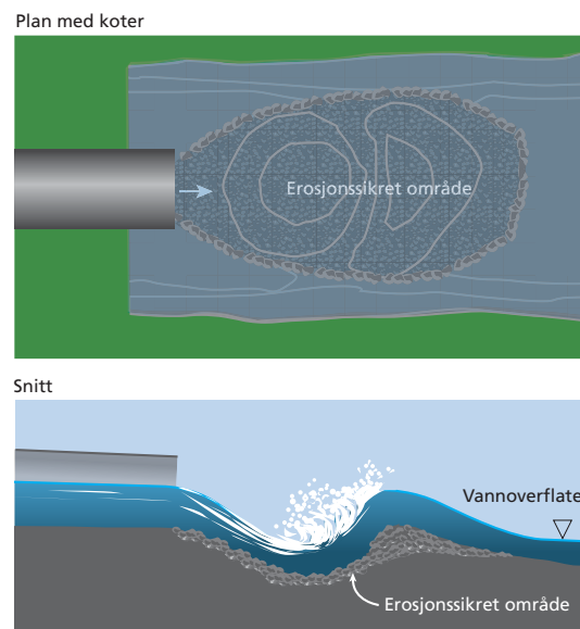
Figur 10.15 Erosjonssikring med steinmasser.
