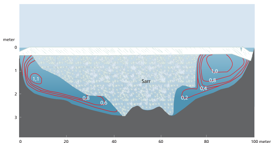
Figur 3.8. Strømforhold og fordeling av sarr og vann i en islagt elv. Kilde: Edvigs V. Kanavin.
