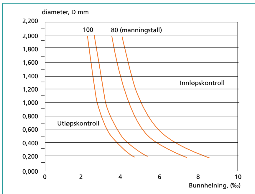
Figur 10.3 Minimumsfall for innløpskontroll: plastrør ( M = 100 ) og betongrør ( M = 80 ). For hver rørtipe gjelder: Høyre kurve: y/D = 0.8 , Venstre kurve: y/D = 0.7 .
