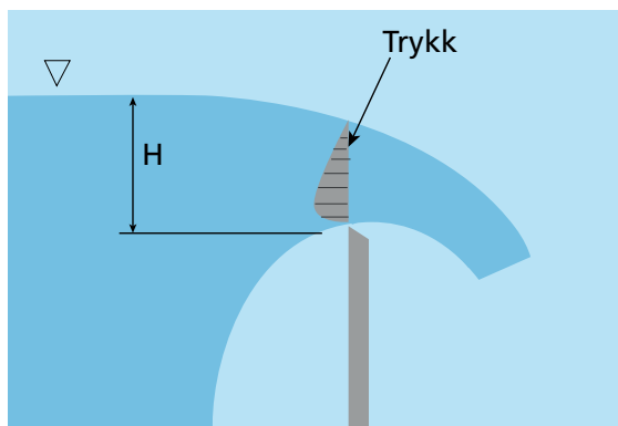
Figur 4.15. Forskjellige overløp
