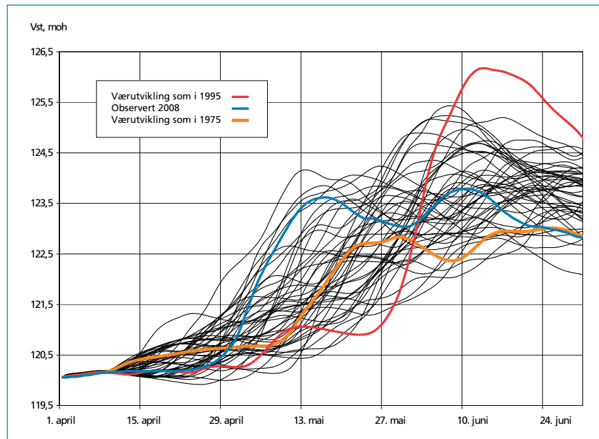
Figur 10. Vannstandsscenarioer for Mjøsa våren og sommeren 2008. Beregningene er basert på scenarioer for tilsig til Mjøsa. Tilsigsscenarioene er beregnet fra hydrologisk tilstand (snømengde, mark- og grunnvannsforhold) i hele Mjøsas nedbørfelt per 1. april 2008. Deretter er de hydrologiske modellene foret med værddata (nedbør og temperatur) fra de siste 50 år, som gir 50 ulike tilsigsscenarioer. Til slutt er dette lest inn i en hydraulisk modell for å beregne vannstandsutviklingen i Mjøsa.
