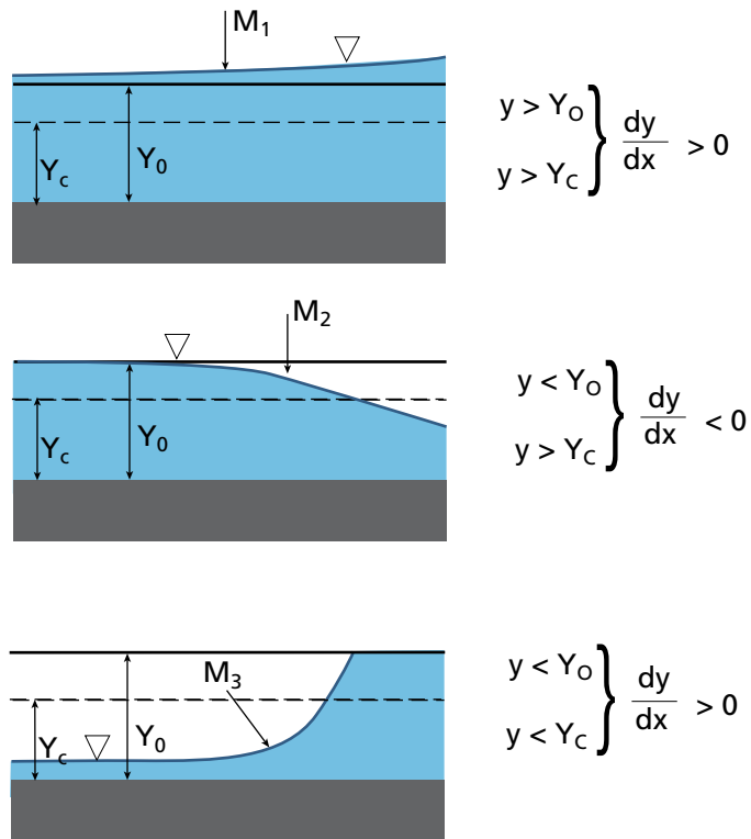
Figur 4.21. Vannlinjer for y_o > y_c
