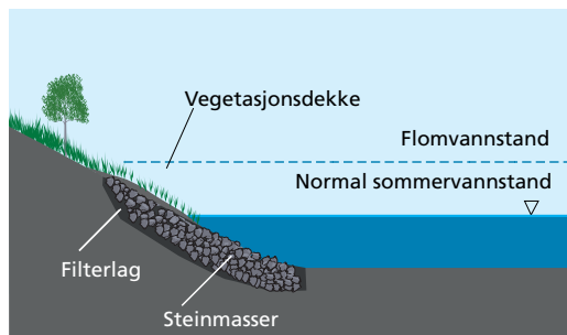
Figur 6.7 Prinsippskisse for erosjonssikring med filterlag og dekklag, se også figur 6.10 og 6.16.
