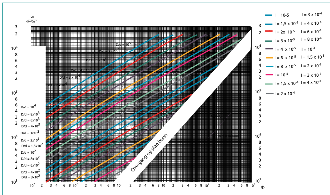
Figur 5.25 Diagram for hastighet og sandtransport (Engelund og Hansen, 1972).
