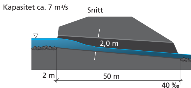
Figur 10.7 Kulvert med innløpskontroll. Strømning type 1.
