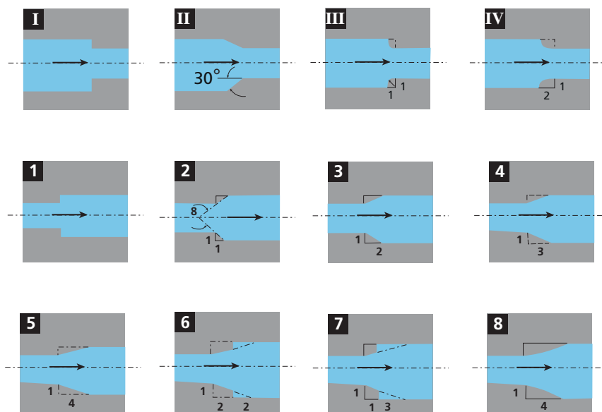
Figur 4.10. Utforming av innsnevringar og utvidelser undersøkt av Formica (1955).
