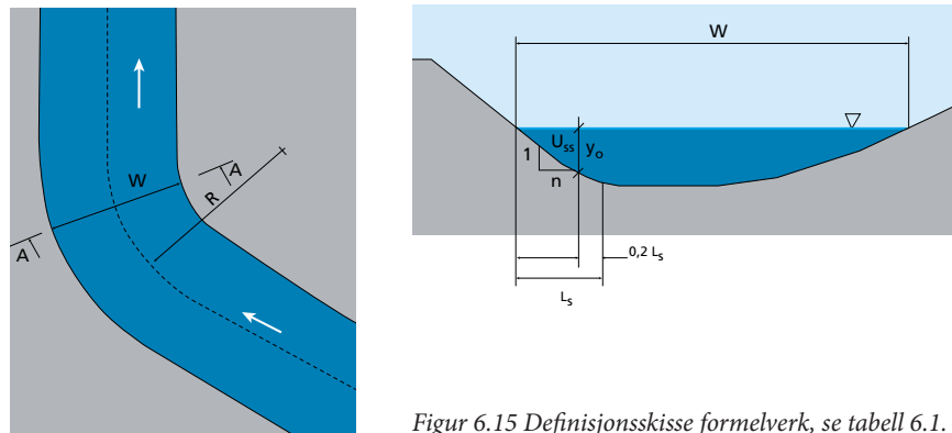
Figur 6.15 Definisjonsskisse formelverk, se tabell 6.1.
