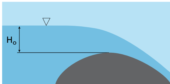
Vanlig overløp C=1,71 Tilsvare likning 4.28
