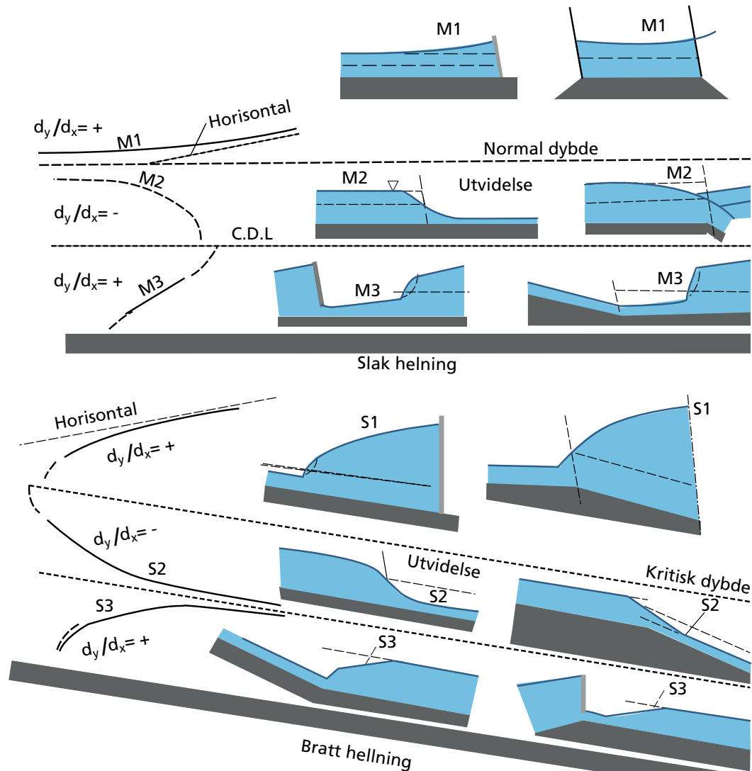
Figur 4.22. Vanlige vannlinjeformer
