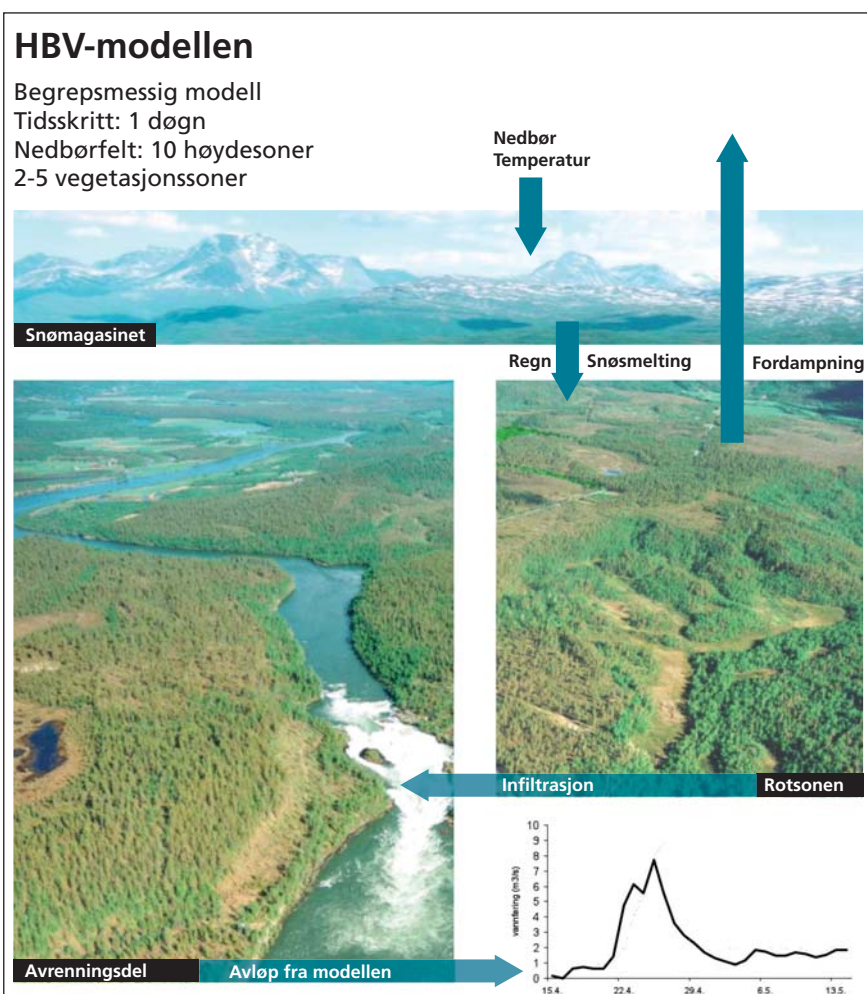
Figur 8a. Øverst, prinsippskisse av HBV-modellen. Inngangsdata er temperatur og nedbør. Snømagasin, fordampning, infiltrasjon og fuktighetsinnhold i rotsonen beregnes i tillegg til vannføring (avrenning). Illustrasjon etter Elin Langsholt, NVE.
