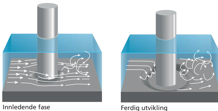
Figur 5.40 Strømmønsteret rundt en sylindrisk pilar og utvikling av erosjonsgrop.
