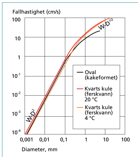
Figur 5.6 Synkehastighet for steinpartikler i vann (tetthet 2650 \text{ kg/m}^3 ).
