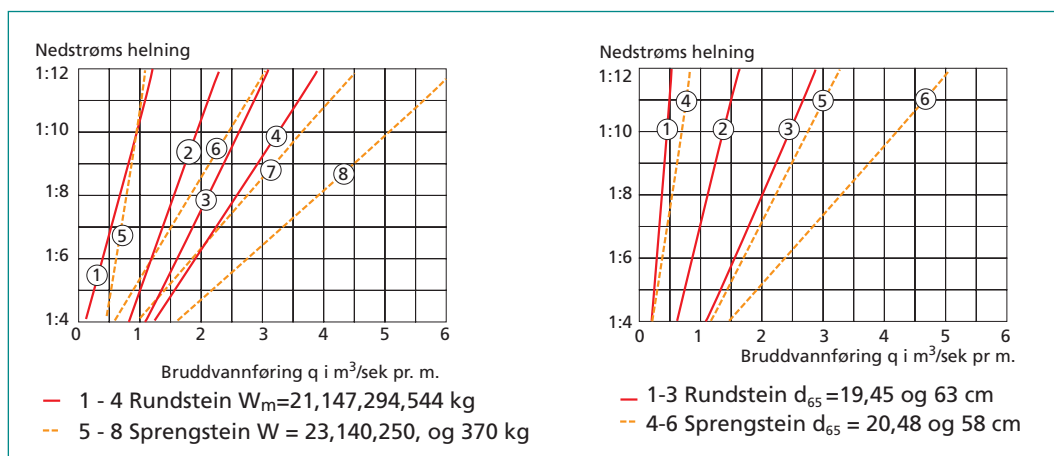
Figur 8.30 Diagrammet til venstre viser bruddvannføring q i \text{m}^3/\text{s}/\text{m} , ensgraderte masser. Diagrammet til høyre viser bruddvannføring q i \text{m}^3/\text{s}/\text{m} , samfengte masser.
