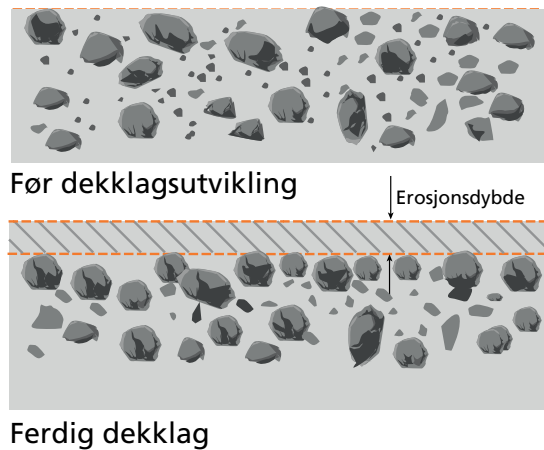
Figur 5.45 Dannelse av naturlig dekklag.
