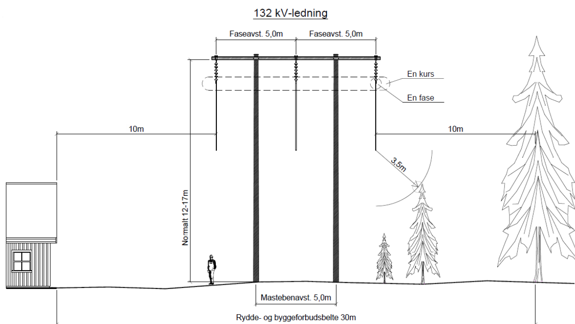
Figur 4-3: Illustrasjon som viser bredden på ryde- og byggeforbudsbeltet ved H-master med 5 m faseavstand.
