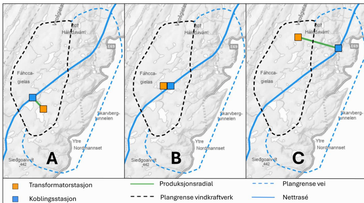
Figur 4-2: A, B, C – tre skisser som illustrerer noen mulige utfall for nettilknytning.
