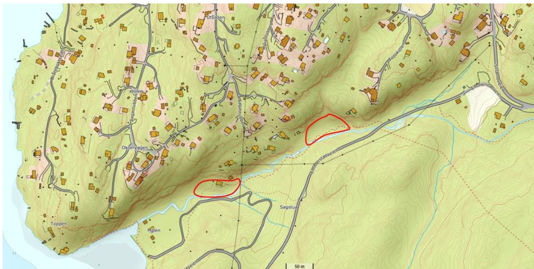
Figur 3: Det er identifisert 2 lokale løснеområder markert i rødt hvor det kan være mulighet for sprøbruddmateriale og terrenghelning som tilsier at det kan gå skred. Utløpsområdet følger bekken nedstrøms.
