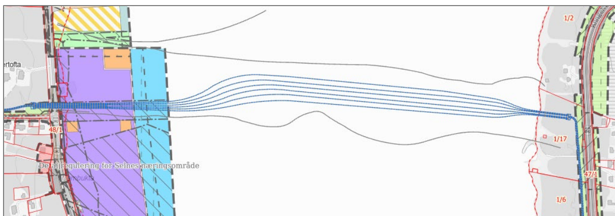
Figur 23 Illustrasjon av omsøkte kabler over Sortlandsundet i vifteformasjon. Eksisterende vann- og avløpsledninger er illustrert med grå linjer. Planlagt utfylt areal på Langøya er illustrert med polygoner.
