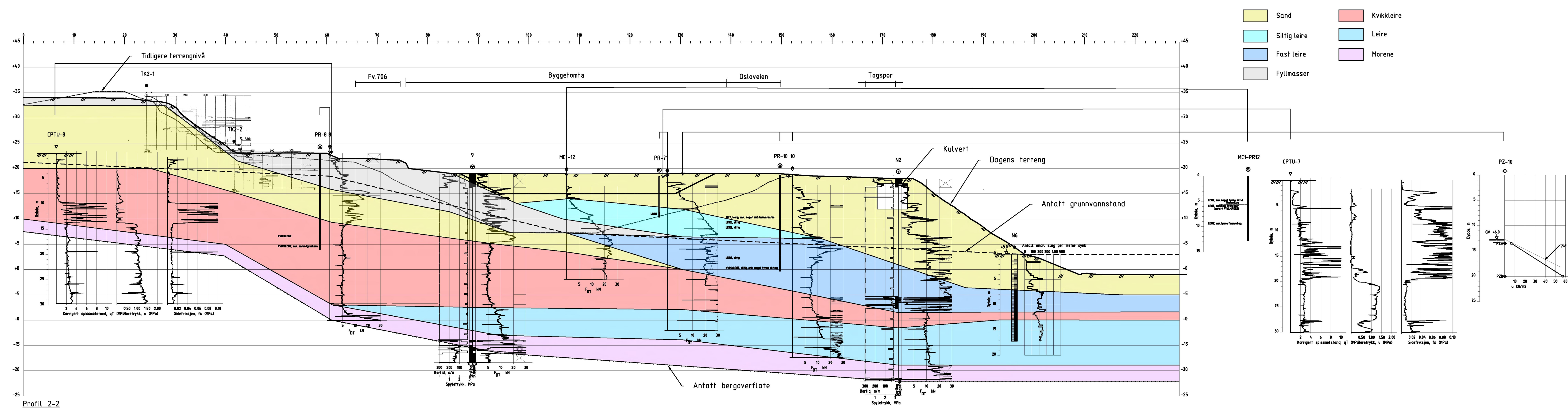
Profil 2-2 1 : 400
