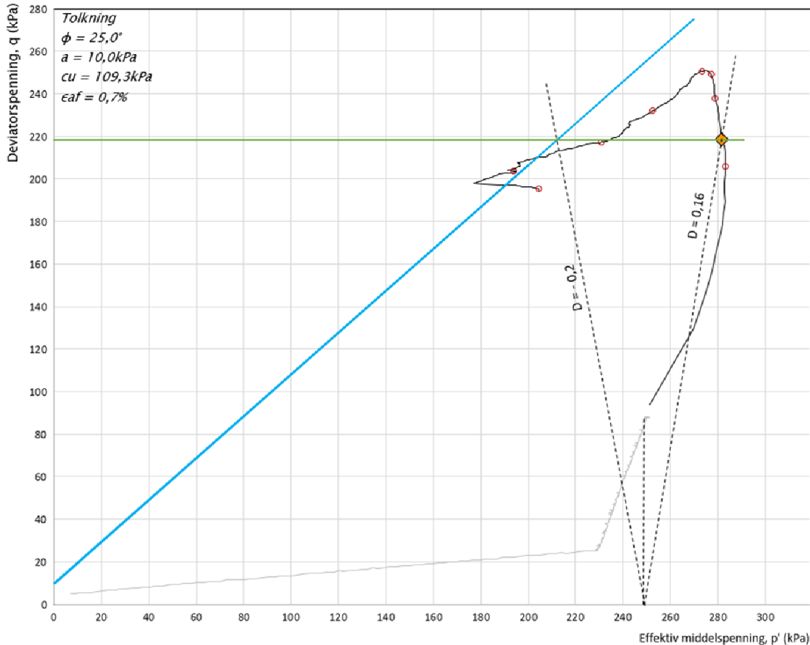
Figur 2 Spenningssti i skjærfase, p' - q plott med tolkning av friksjonsvinkel og attraksjon (Bp.10, dybde 18,43 m under terreng)
