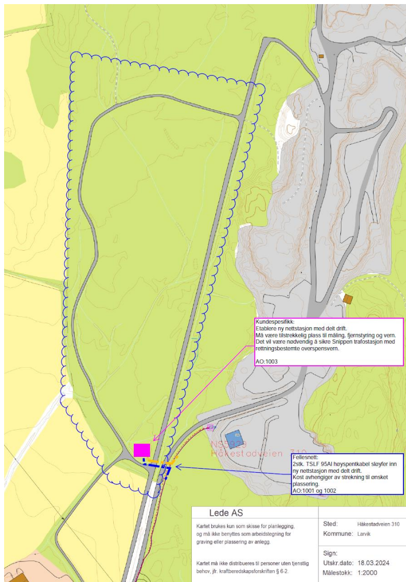
Figur 2-5: Skisse for planlegging av nettilknytning fra Lede AS
