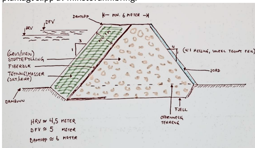
Figur 1. Skisse av plan for damkonstruksjon.
