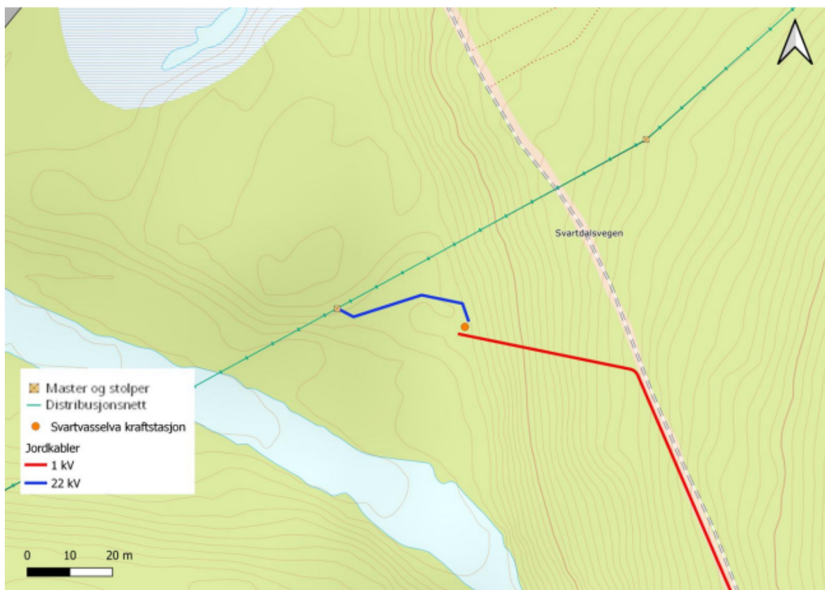
Figur 1: Svartvassselva kraftverk tilknyttes overliggende nett via en omtrent 35 meter lang 22 kV jordkabel. Jordkabelens trasé er markert med blå strek. Rød strek viser lavspentkabel langs rørgata. Kilde: Småkraft sin søknad av mars 2025
