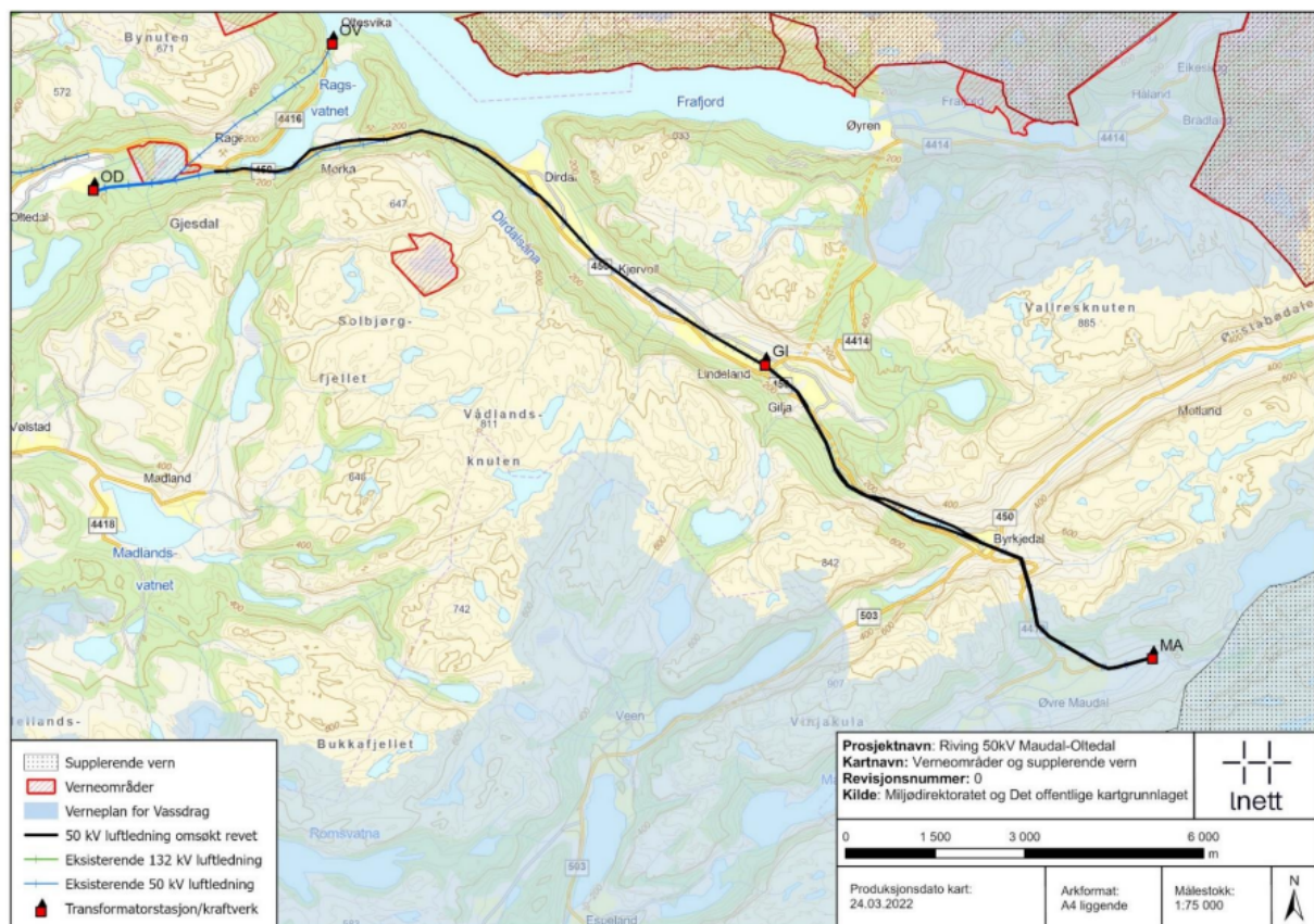
Figur 1: Ledningene som er omsøkt revet er vist med sorte streker. Blå strek ved Oltedal viser ledning som vil bli stående. Kilde: Søknad av 28. juni 2024
