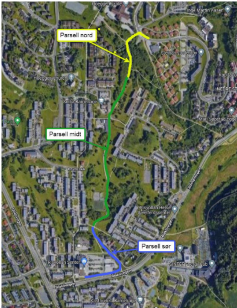
Figur 1: Figuren viser planlagt trasé for nytt hovedrørnett til Steinan.
