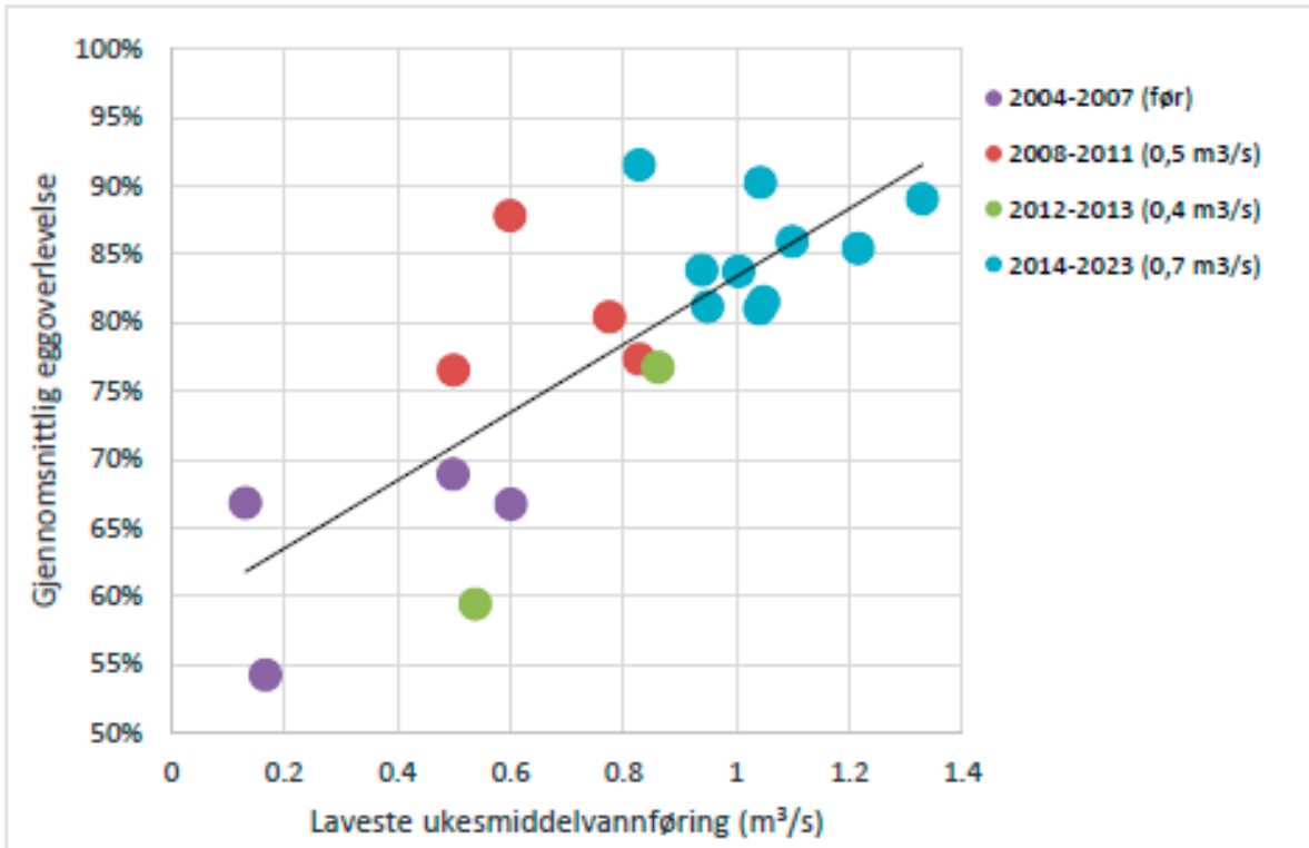
Figur 6.3: Sammenhengen mellom laveste ukemiddelvanntføring om vinteren og gjennomsnittlig eggoverlevelse i registrerte gytegrøper påfølgende vår. Figuren er hentet fra Skoglund m.fl., 2023a.
