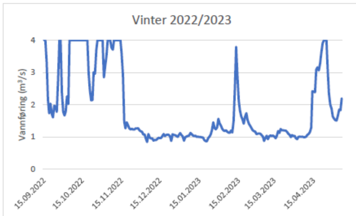
Figur 6.2: Vannføring (døgnmiddel) ved Blåsteinen, Bjoreio, i perioden 15.09.2022 til 07.05.2023. Kurven viser bare vannføringer < 4 m 3 /s. (Figuren er hentet fra Skoglund m.fl., 2023a).
