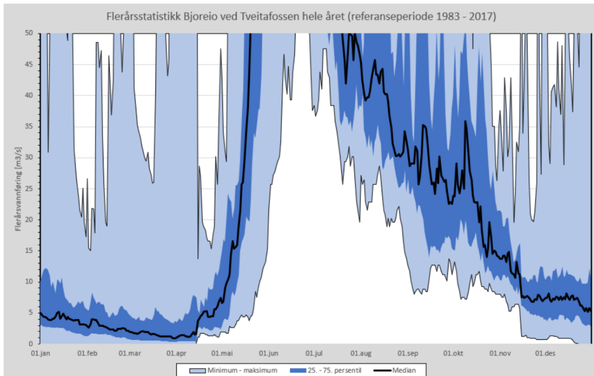
Figur 6.1: Flerårsstatistikk for uregulert vannføringer under 50 m 3 /s i Bjoreio ved Tveitafoss i perioden 1983 til 2017. (figuren er hentet fra Statkrafts tilleggsutredning, dok #49).
