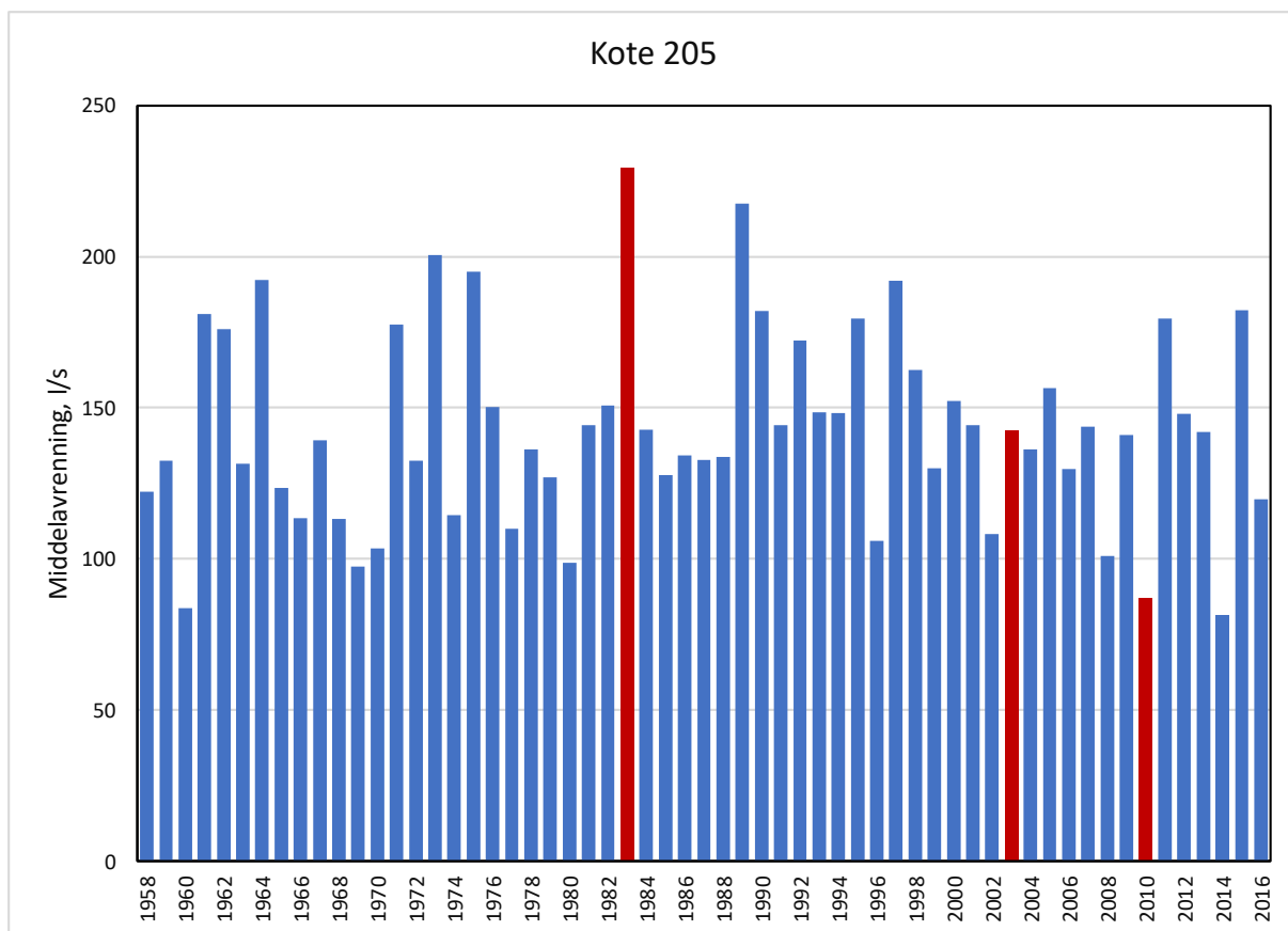
Figur 5. Plott som viser variasjoner i middelvannføring fra år til år (1958-2016). Røde søyler indikerer vått år (1983), middels år (2003) og tørt år (2010). Årsmidler skalert etter målestasjon 138.1 Øyungen. 16
