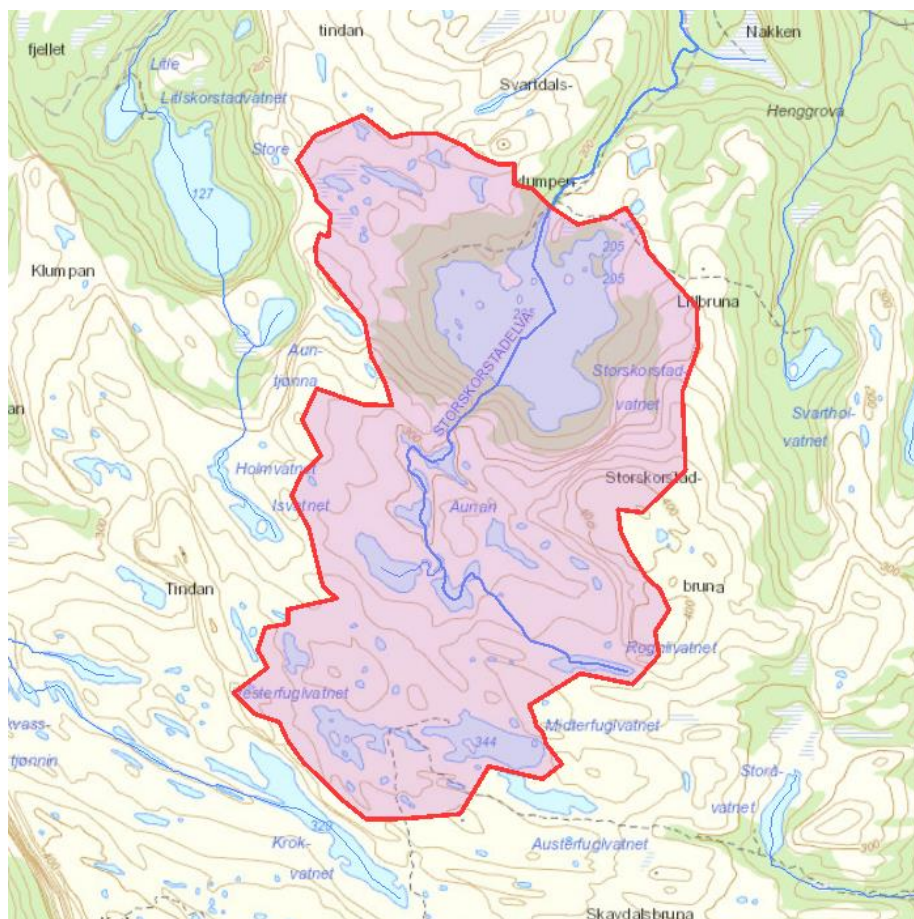
Figur 1B. Kart som viser nedbørfeltet til settefiskanleggets inntakspunkt på kote 205, generert i NEVINA.
