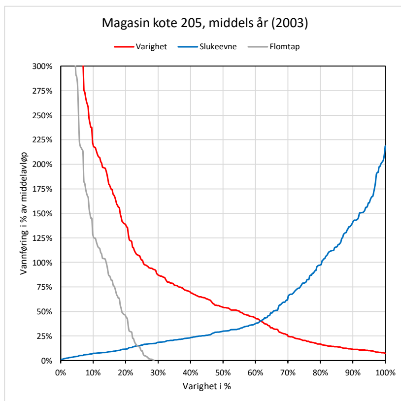
Figur 11. Varighetskurve, kurve for flomtap og for tap av vann i lavvannsperioden (år). Slukeevne = middel vannuttak for året, 22,8 l/s.
