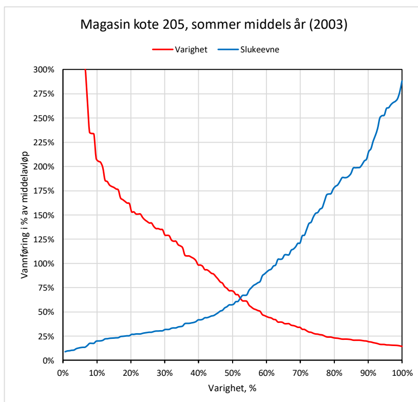
Figur 9. Varighetskurve for sommersesongen (1/5 – 30/9). Slukeevne = middel vannuttak i perioden, 30 l/s.
