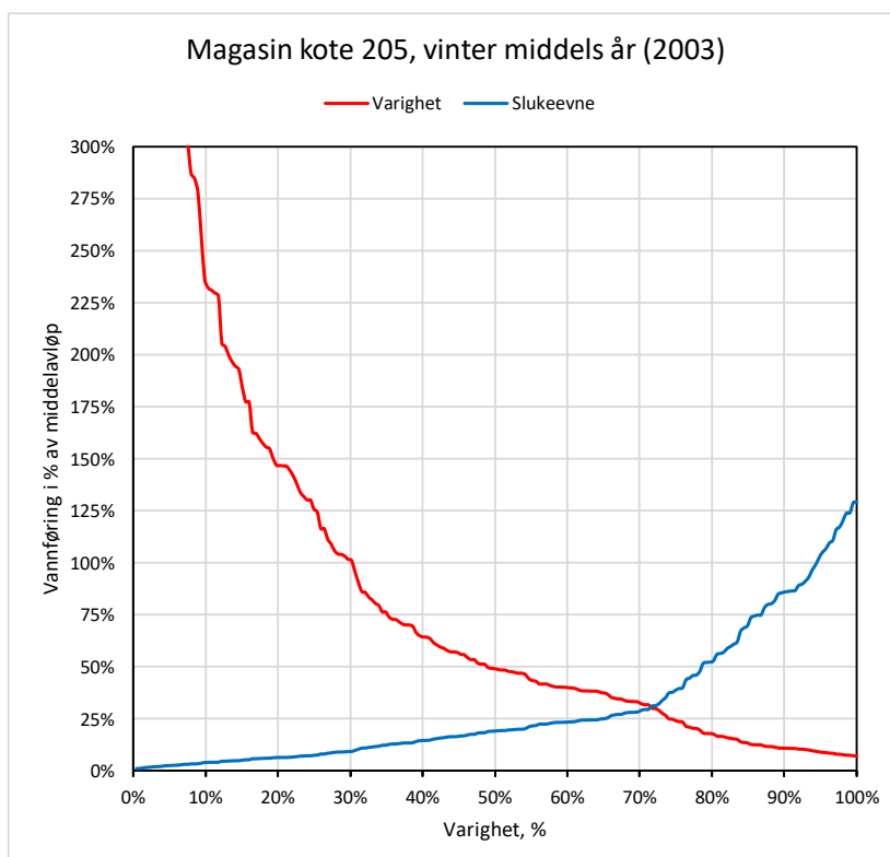
Figur 10. Varighetskurve for vintersesongen (1/10 – 30/4). Slukeevne = middel vannuttak i perioden, 17,6 l/s.
