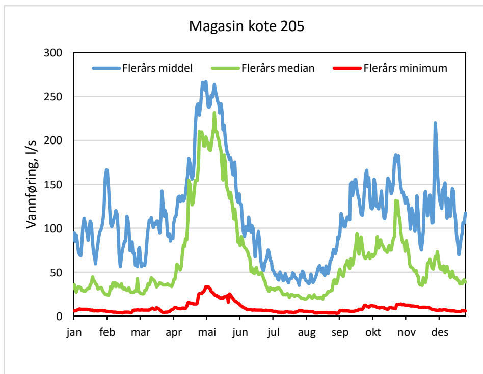
Figur 3. Plott som viser sesongvariasjon i middel/median- og minimumsvannføringer gjennom året, (døgndata). 14
