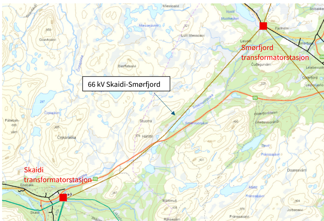
Figur 1: Trasé for 66 kV Skaidi-Smørfjord (brun linje). Kilde: NVE Atlas
