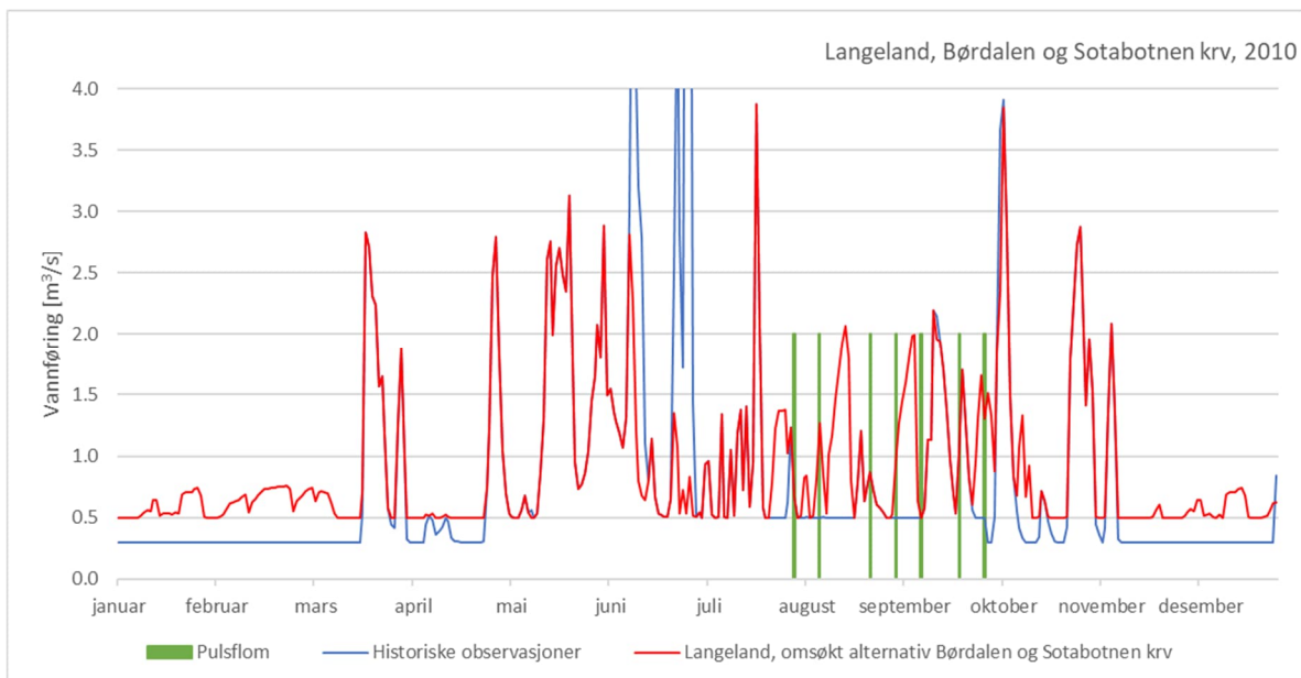
Figur 5-49 Pulsfloam ved Langeland for 2010, omsøkt alternativ Børdalen og Sotabotnen krv
