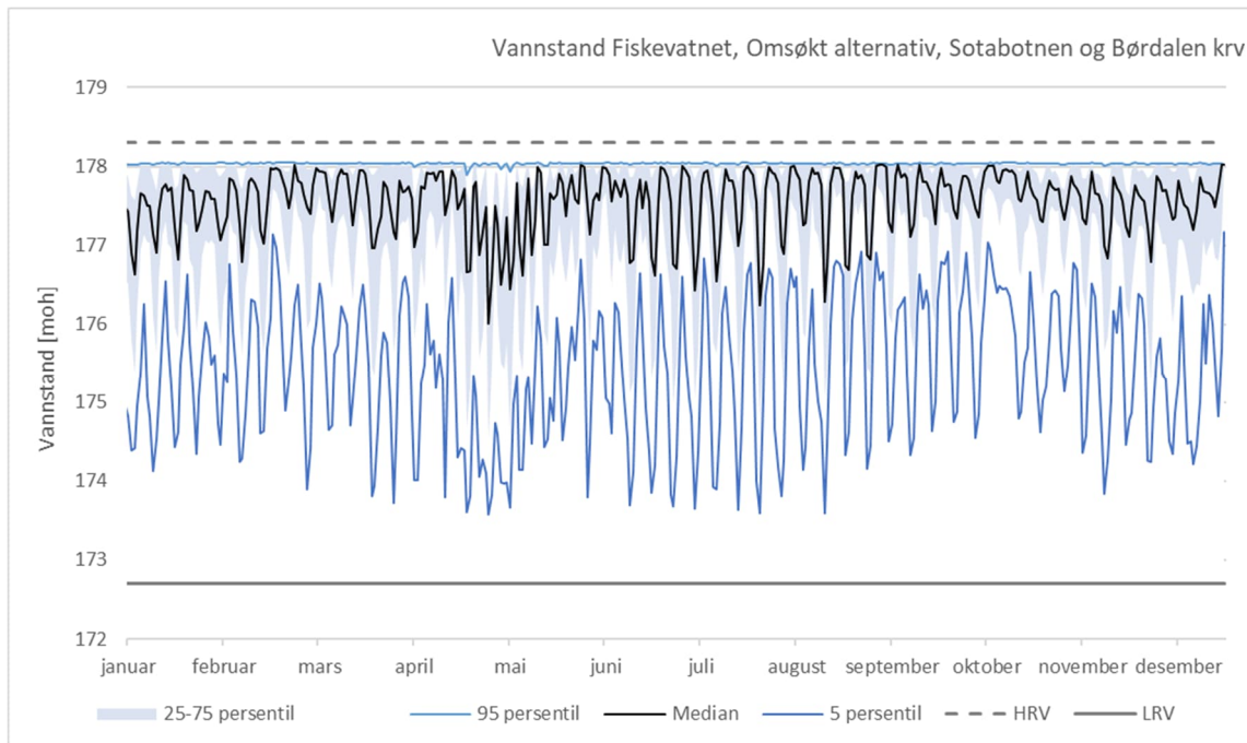
Figur 5-32 Persentilcurver for vannstand i Fiskevatnet ved omsøkt alternativ
