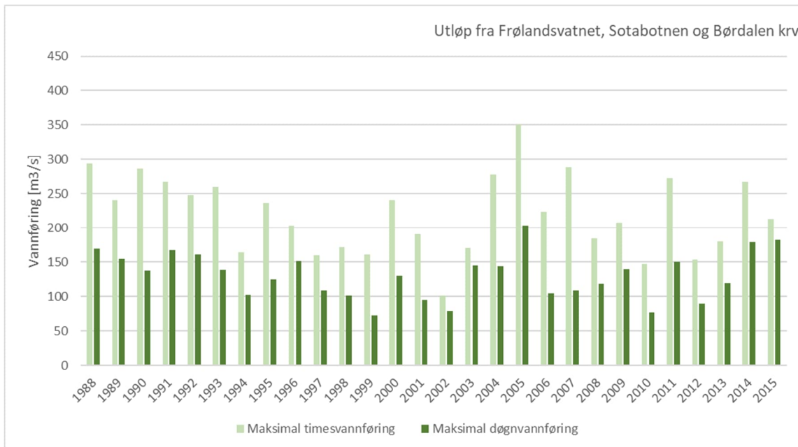
Figur 9-7 Maksimal flomstørrelse pr år etter omsøkt alternativ, Sotabotnen og Børdalen kriv
