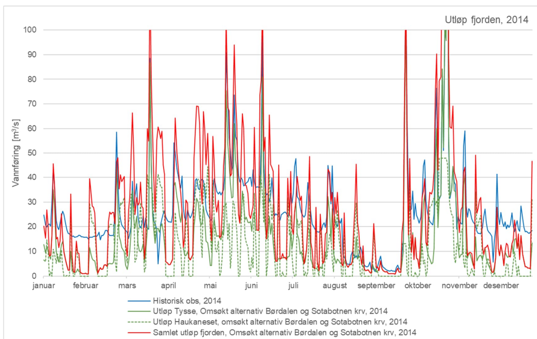
Figur 5-76 Vannføring til fjorden, døgn gjennomsnitt, 2014.
