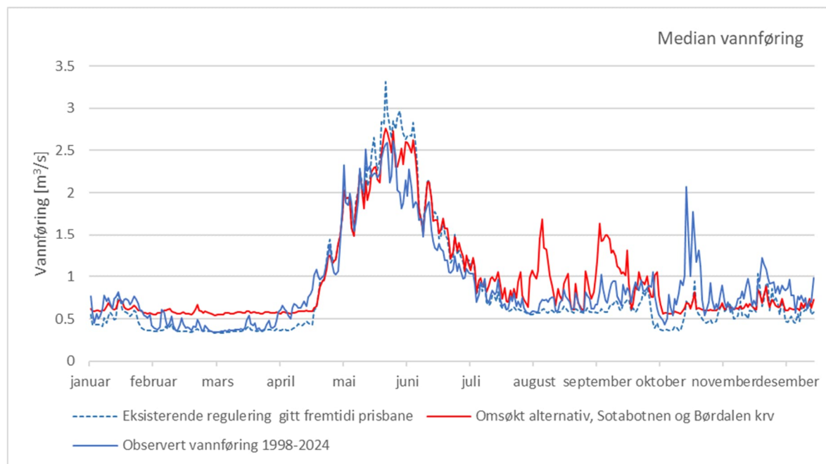
Figur 5-52 Medianvannføring ved utløp av Storelva i Frølandsvatnet, observert vannføring, eksisterende regulering gitt fremtidig prisbane og etter omsøkt alternativ
