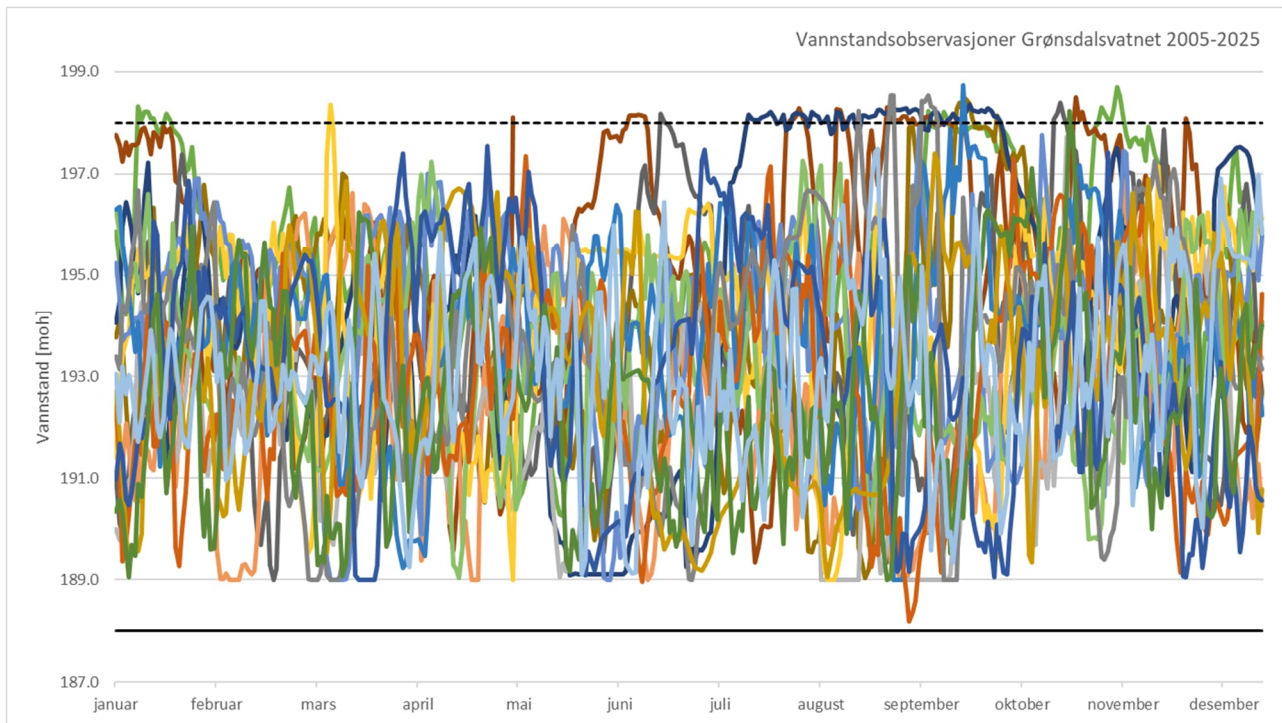
Figur 5-26 Observert vannstander i Grønsdalsvatnet mellom 2005-2024
