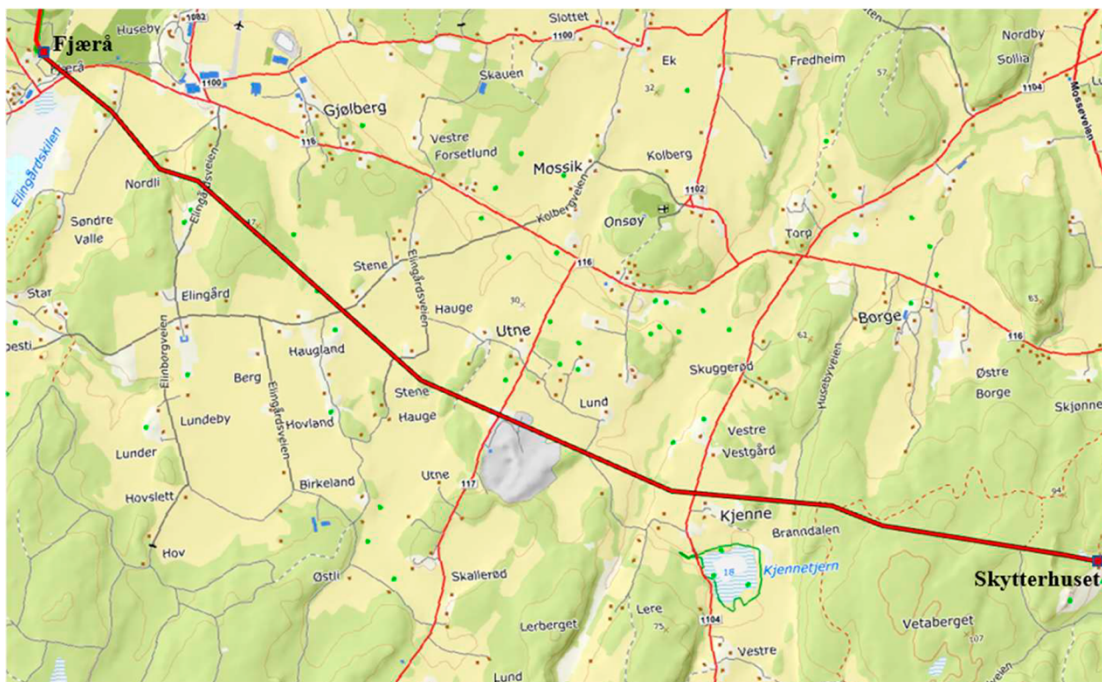
Figur 4: Dagens ledningstrasé Fjærå–Skytterhuset, hvor Elvia søker om å strekke nye 47 kV ledninger på eksisterende fagverksmaster. Kilde: Elvia sin søknad.
