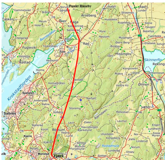
Figur 2: Konsesjonssøkt trasé for ny 132 kV luftledning Huseby–Fjærå med rød strek. Kilde: Elvia sin søknad.
