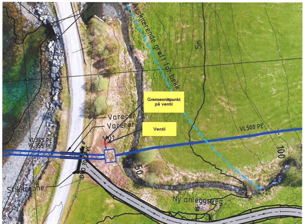
Situasjonsplan
