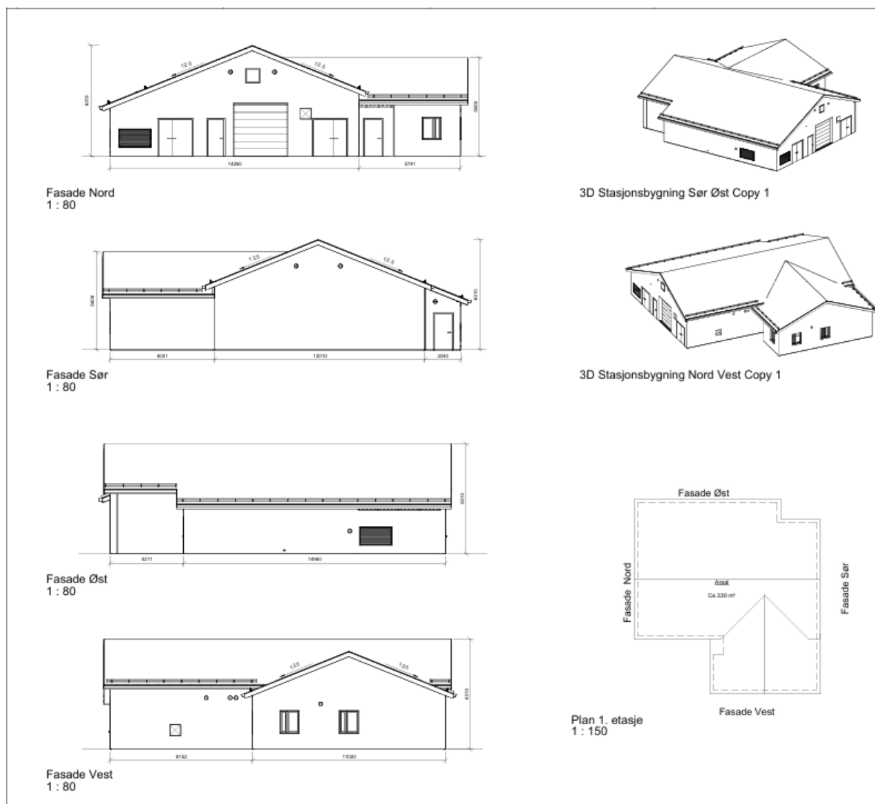
Figur 2: Fasadetegning av stasjonsbygget fra forskjellige vinkler.
