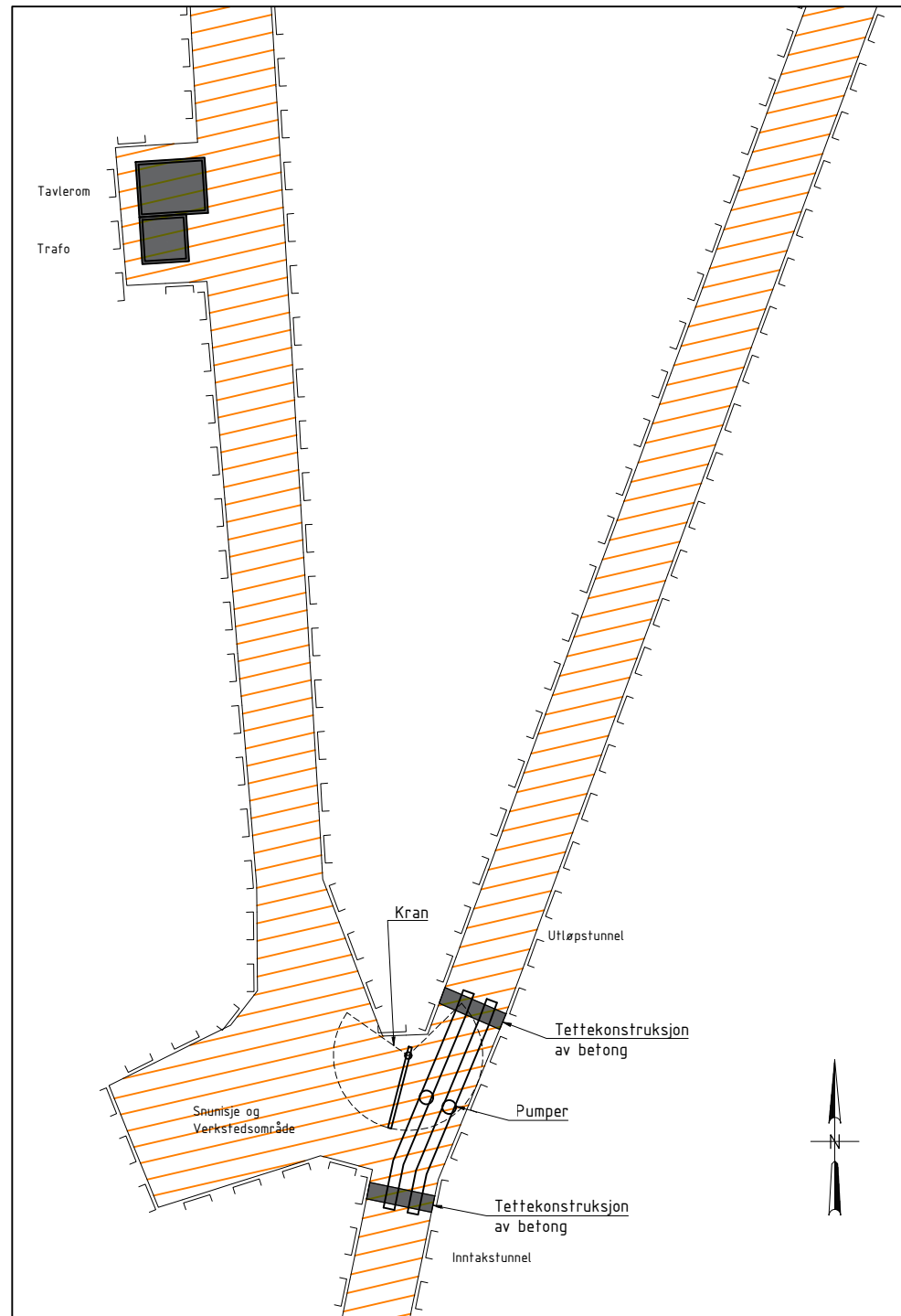
Plan. Pumpestasjon i berg
