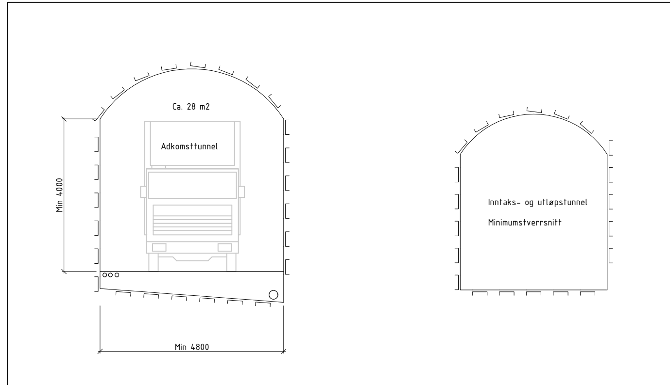
Typiske snitt bergtunneler
