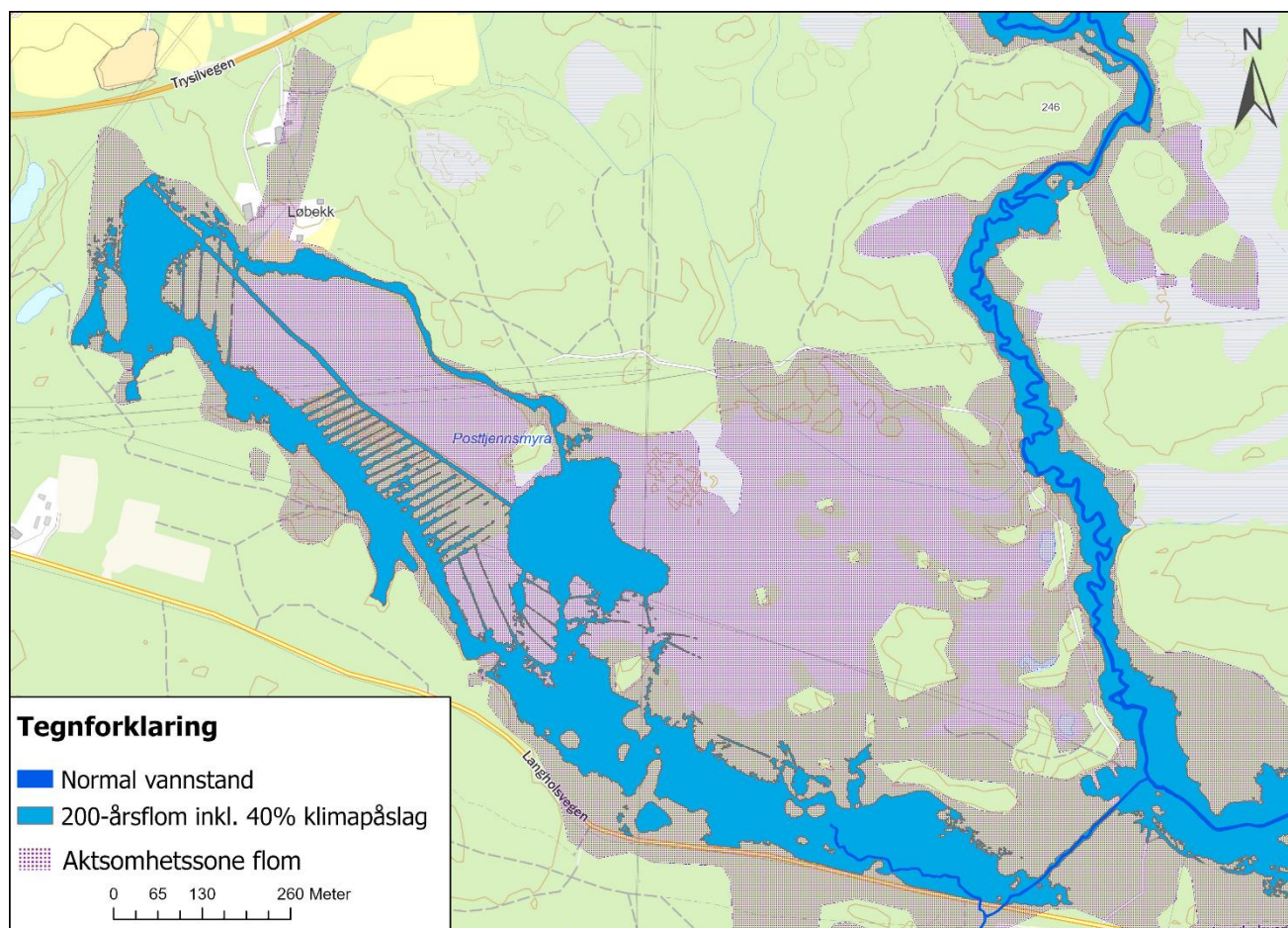
Figur 7. Beregnet flomutbredelse for Nistilen og bekk fra Posttjernsmyra i forhold til NVEs aktsomhetskart for flom.
