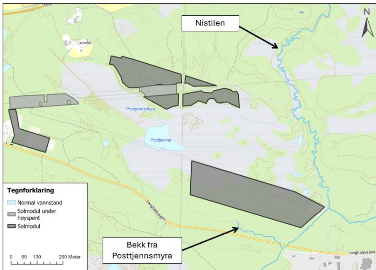
Figur 1. Teknisk plan for solkraftverk. Øst for anlegget renner elva Nistilen. © Kartverket.
