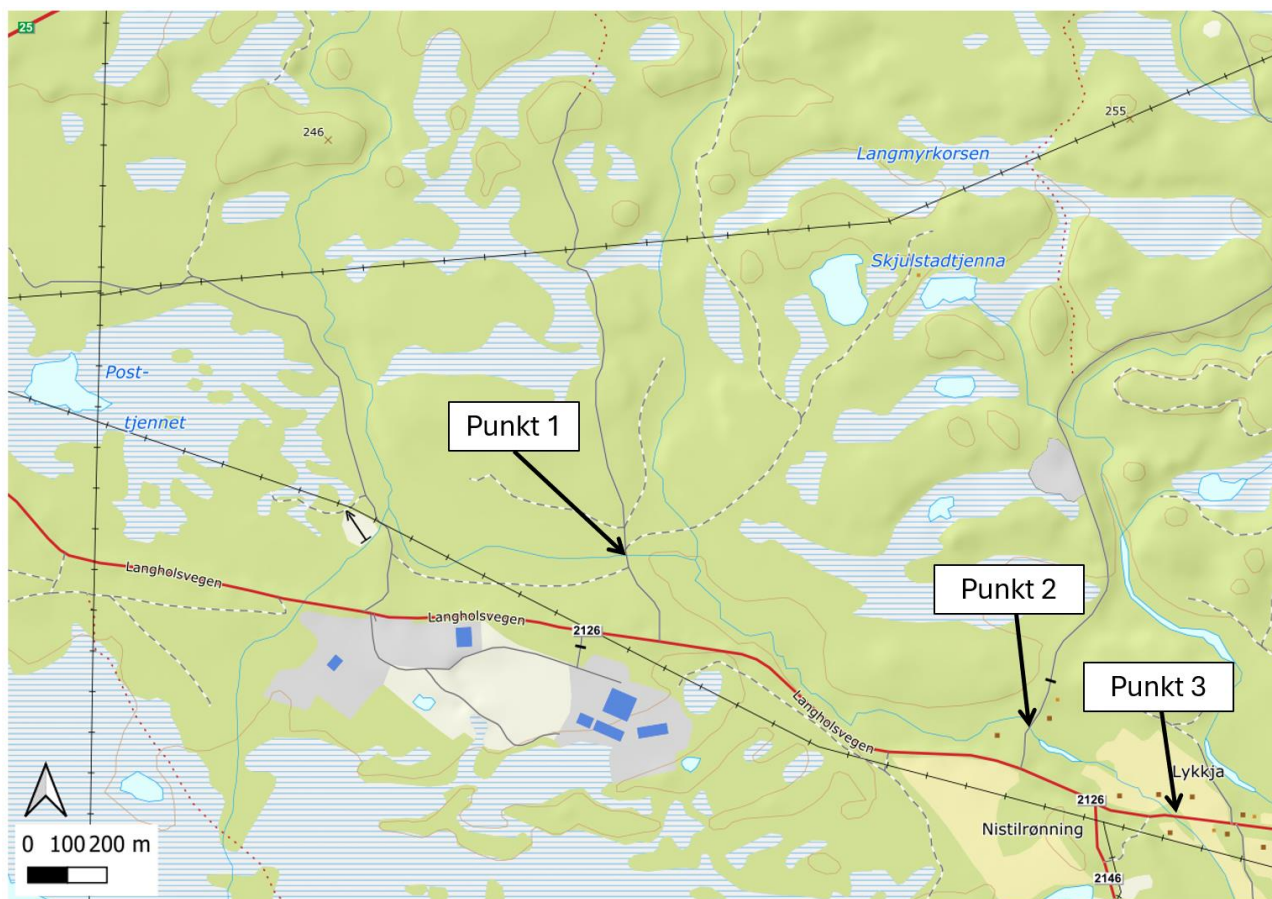
Figur 6. Krysningspunkt under veg for Nistilen langs beregningsstrekingen.
