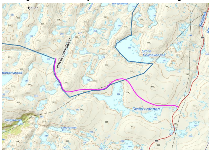
Govva 5. Evttohuvvon sisabeassangeidnu bieggafápmorusttegi Fg888:us, merkejuvvon čuvgesruksesiin .
