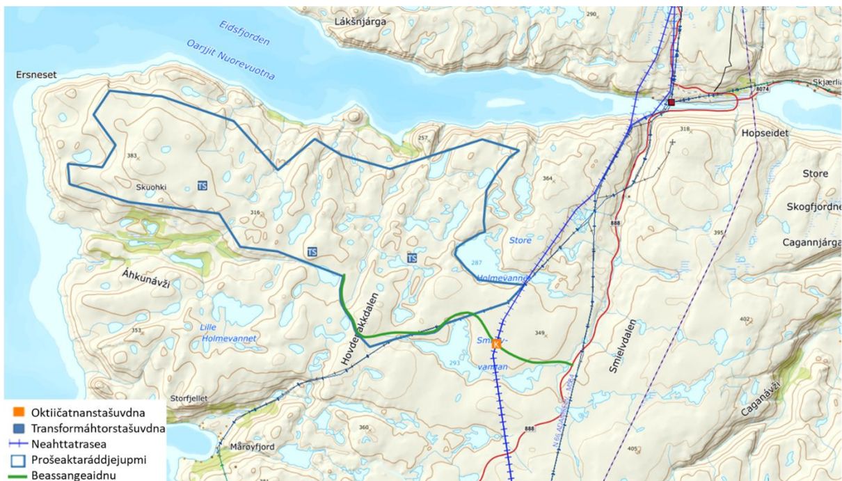
Govva 8. Evttohuuvon stašuvdnačovddus Lágesvuona bieggafápmorusttegii, gaskaboddosaš transformáhtorstašuvnnaid sajusteapmi.
