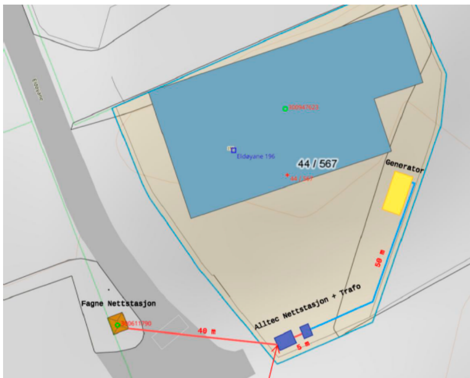
Figur 1 – Generator, kabelanlegg og nettstasjon + trafo planlegges inne på eiendommen.
