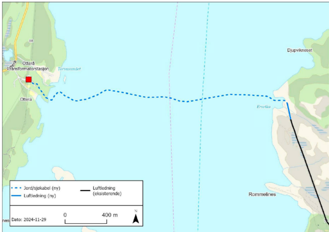
Figur 2-1 Omsøkt 66 kV (132 kV) sjøkabel Reksteren/Tysnes til Otteråi/Austevoll.
