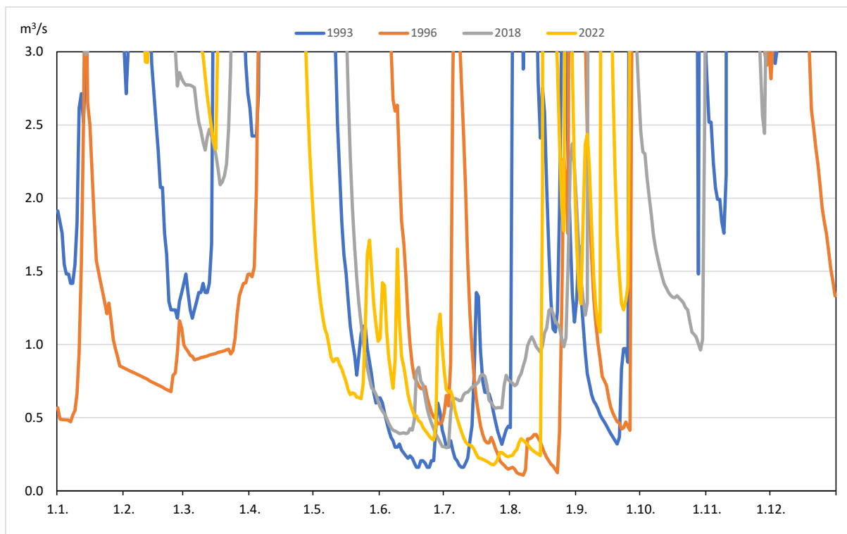
Figur 2: Beregnede vannføringer til Søndeled inntaksdam i fire tørre år. I den nederste figuren er bare vannføringer lavere enn 3 m 3 /s vist slik at detaljer i lavvannsperioder kan vises.
