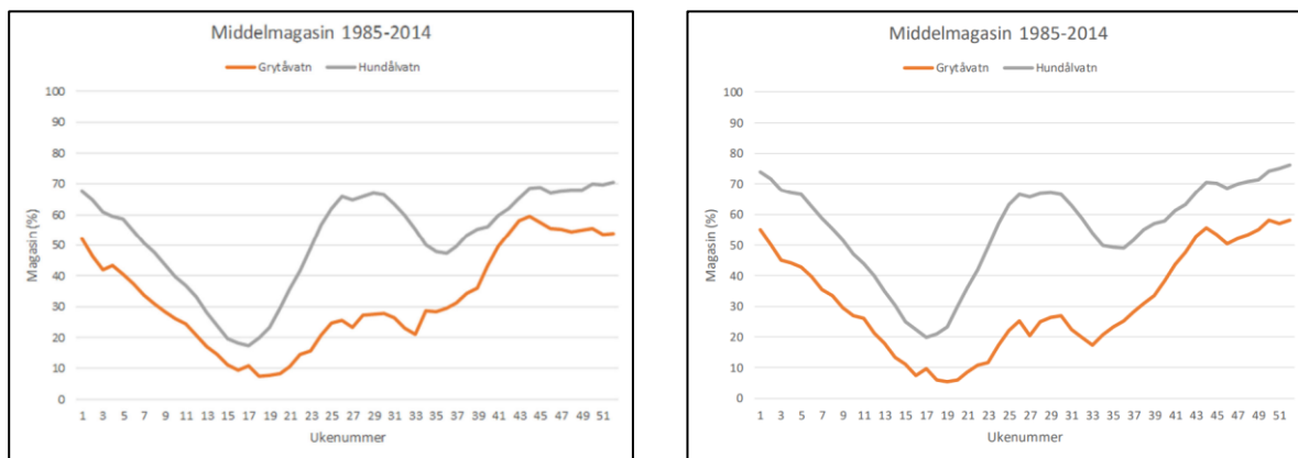
Figur 2: Magasinkurve Grytåga kraftverk med dagens slukeevne (venstre) og økt slukeevne (høyre).
