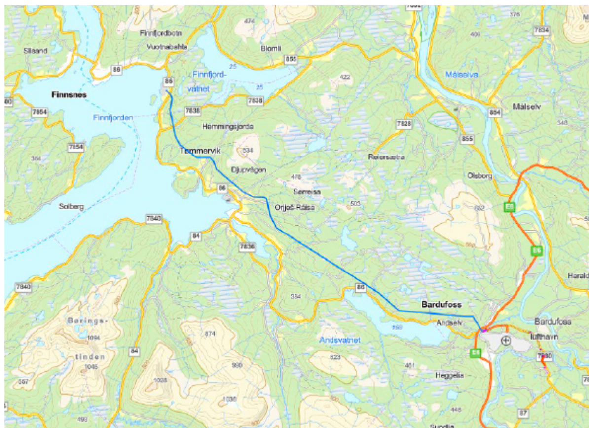
Figur 2-2. Blå strek viser den konsesjonsgitte linjetrasé mellom Bardufoss og Finnjordbotn. Kilde NetBas.
