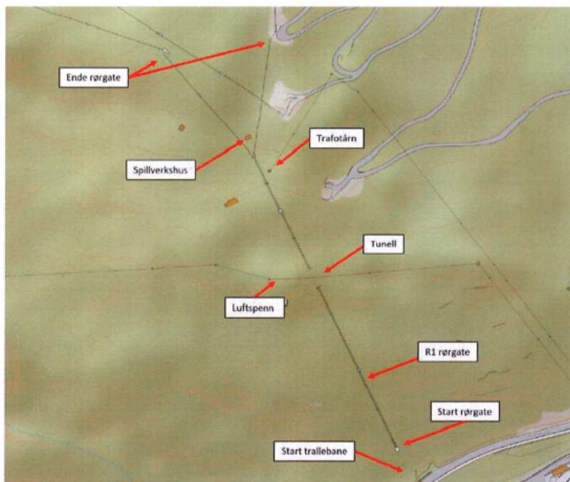
Figur 1-2 Oversikt rørgate, spillverkshus og trafotårn i K1. Trapp og trallebane følger same trasé
