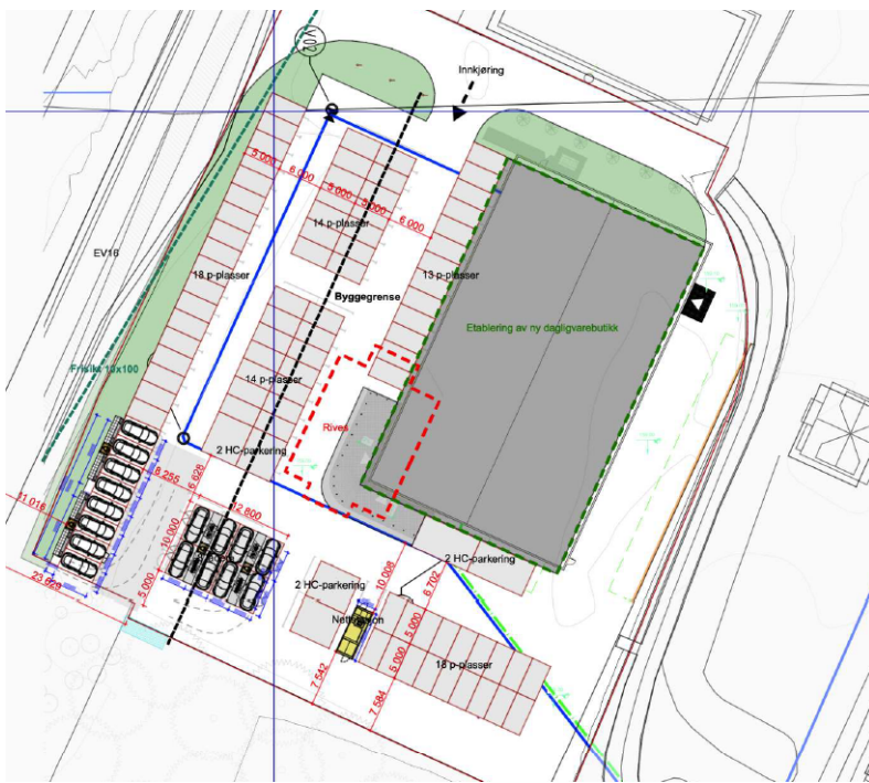
Figur 2 Nettstasjonen, vist i gult, skal plasseres på parkeringsplass i Ådalsveien 149 i Hallingby i Ringerike.
