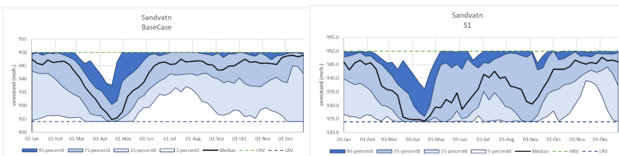
Figur 3-12 Sammenligning av magasinfyllingskurver av Sandvatnet for et tørt år, et middels år og et vått år etter utbygging av Kvanndal 2B og Suldal 2B, sammenlignet med historiske data og simulert BaseCase. Kurven «S1» gjelder utbygging av Kvanndal 2B + Suldal 2B.
