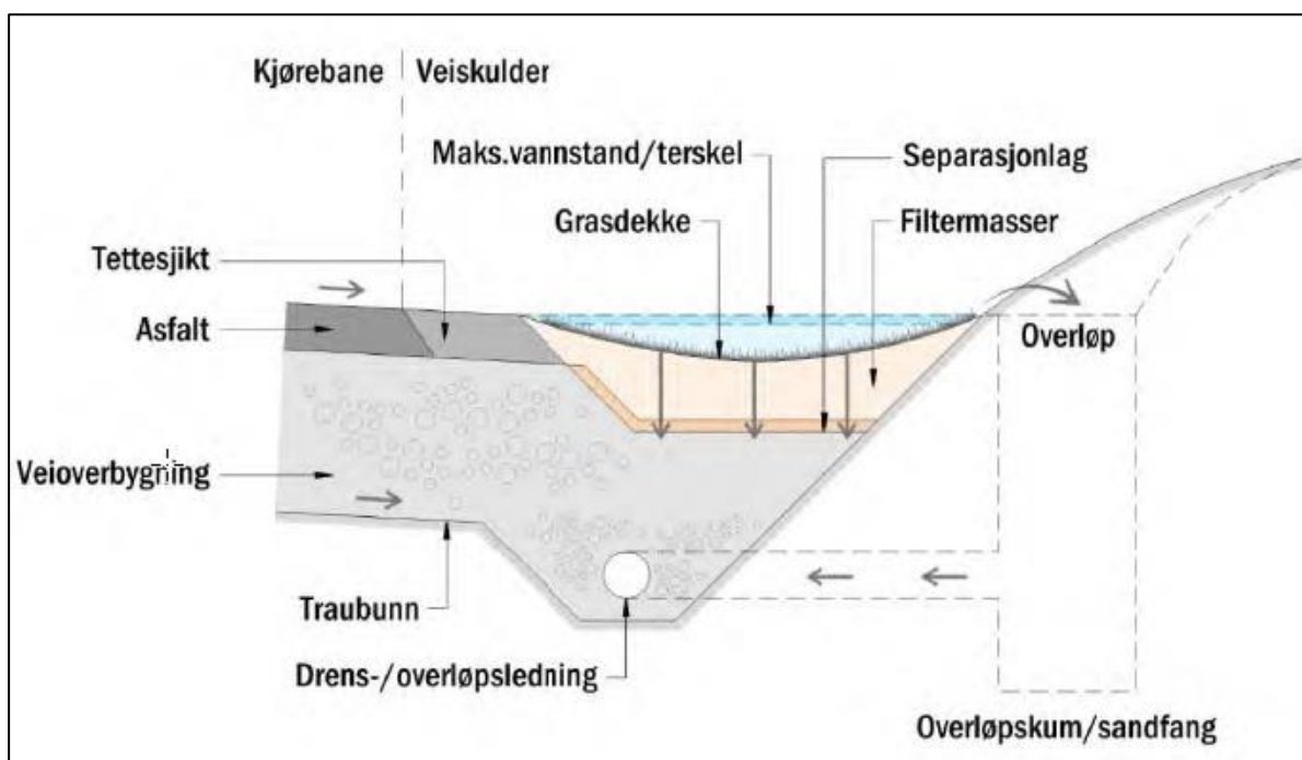
Figur 20. Prinsipp for infiltrasjonsgrøft i jordskjæring
