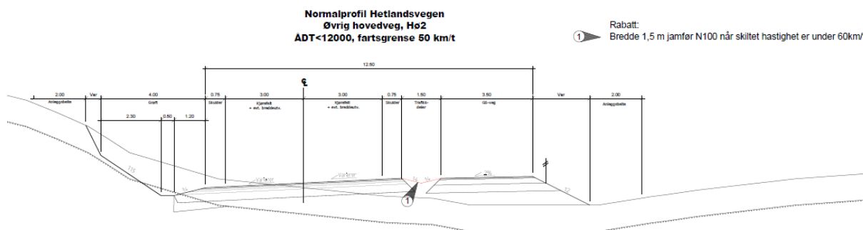
Figur 21 Normalprofil Hetlandsvegen. Tegning F101 som er inkludert i vedlegg 13.
