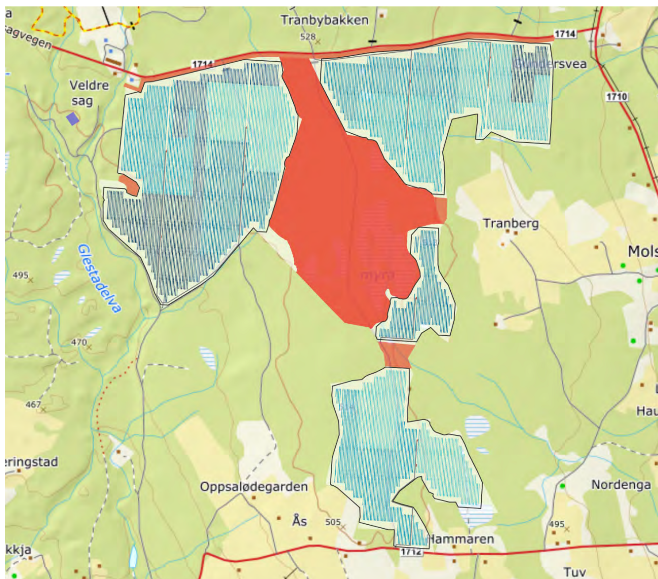
Figur 2 Foreløpig layout for Tranmyra agrivoltaiske solkraftverk. kilde; Kilden.nibio.no
